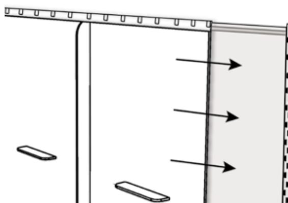
Een Tree Root Guiding paneel in de vorm van een 90° graden hoek. De hoek is aan beide zijden gekoppeld aan een in- en uitschuifbaar Tree Root Guiding paneel zodat deze ten alle tijden voor iedere afmeting plantgat toepasbaar is.
